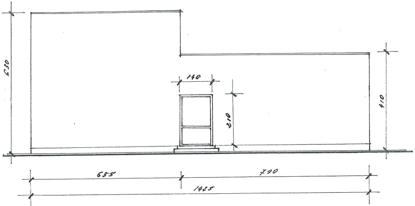
Elewacja boczna – prawa
